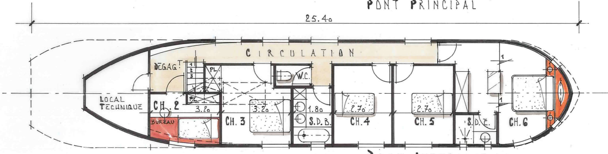
PONT INFÉRIEUR
