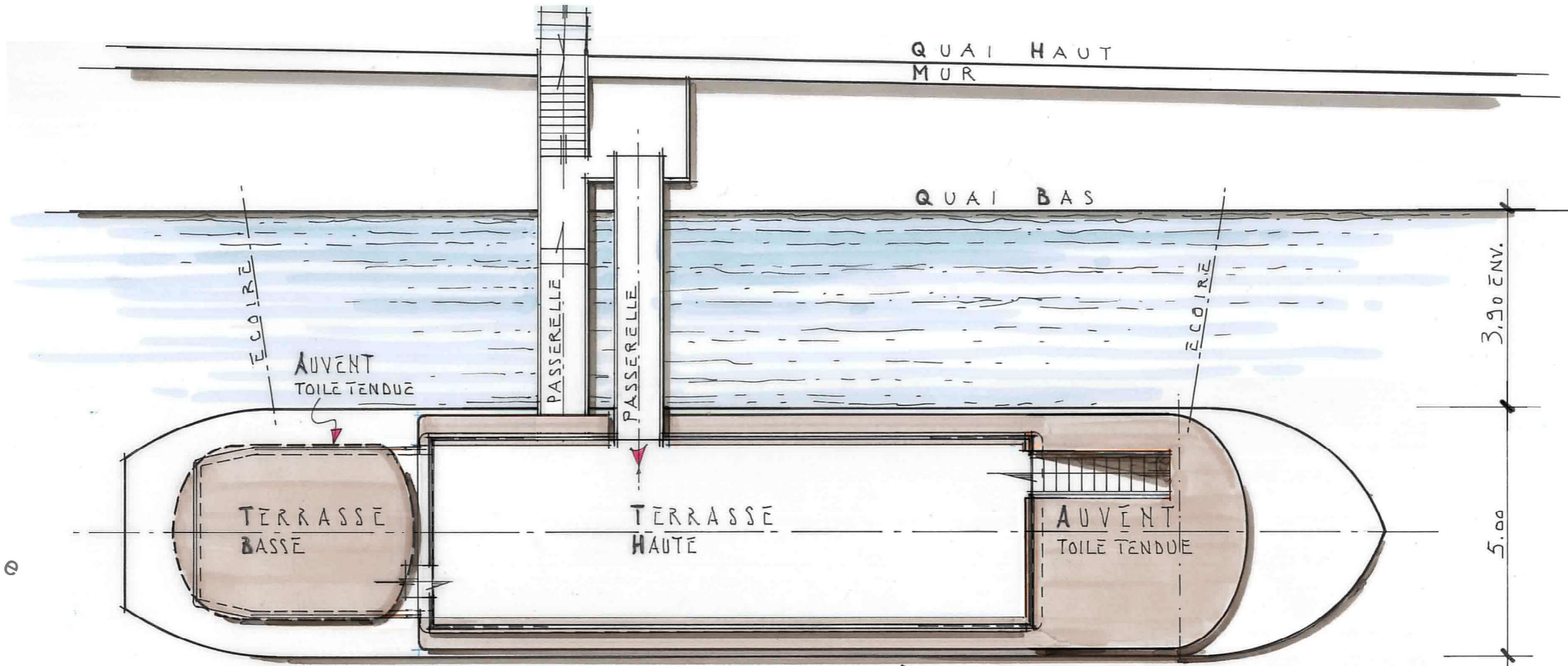
PONT TERRASSE Echelle 1/100
